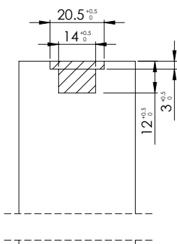
SECTION B-B SCALE 1 : 2
