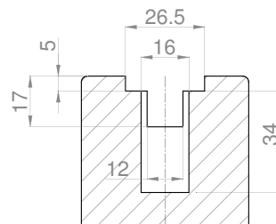
Section D-D
