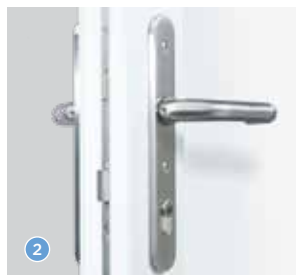
Falle-Riegelbereich mit Auslöser
