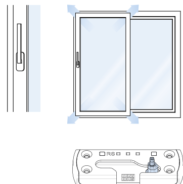
Porte coulissante entrebâillée jusqu'à 6 mm
