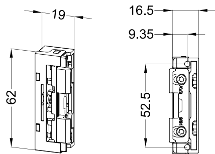
Dimensioni principali con funzione di passaggio (d)
