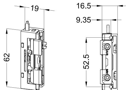
Dimensioni principali del fermo a giorno (a+b)
